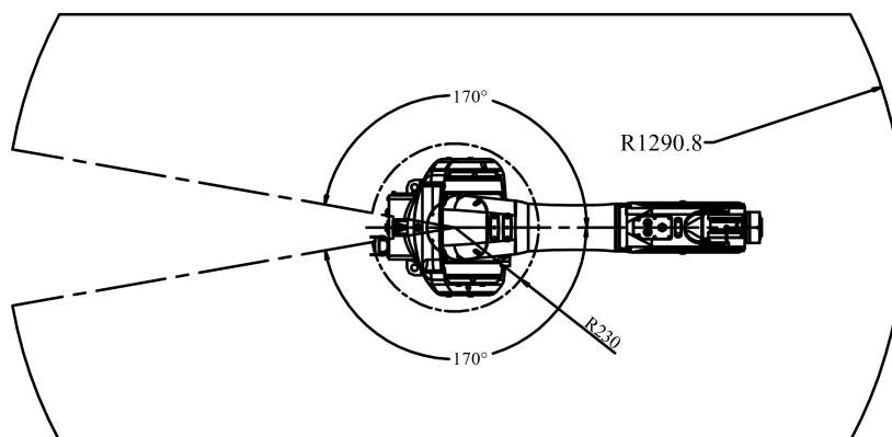
图 2-5 机器人工作空间图
