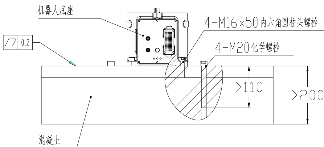
图 3-3 地面安装
