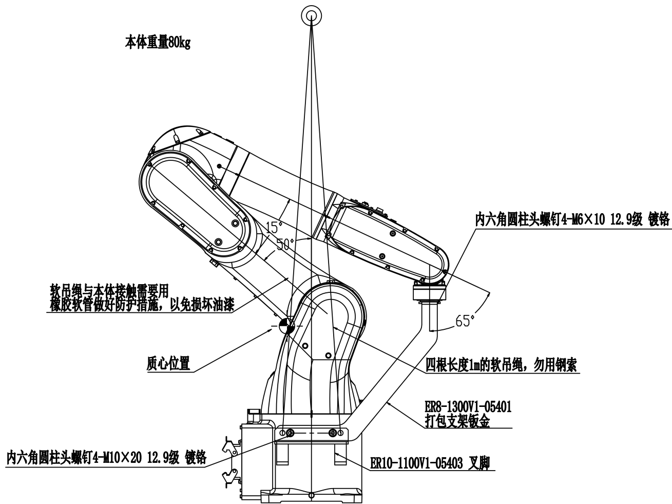
图 3-1 吊装搬运示意图
