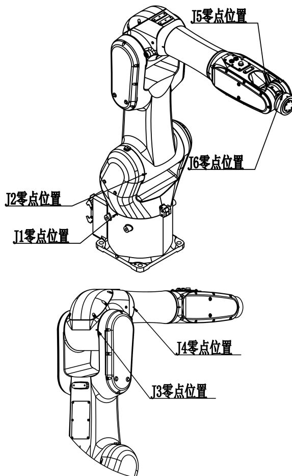
图 4-2 机器人零点位置图
