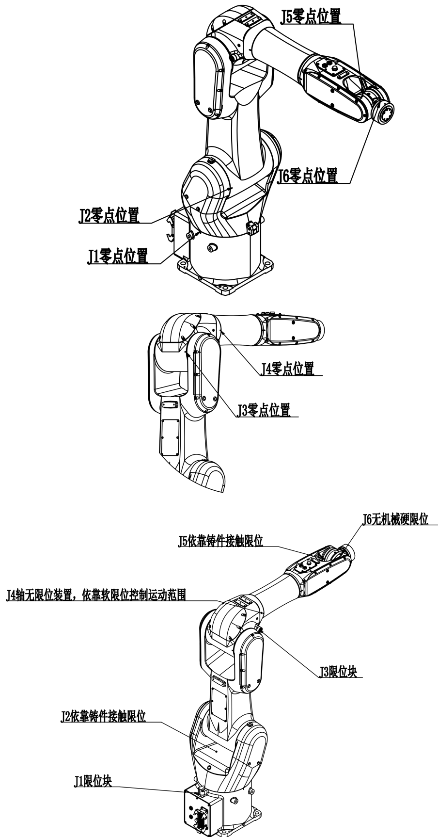
图 2-4 机械硬限位位置及零标位置
