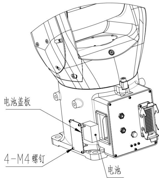
图 4-3 机器人电池组位置图
