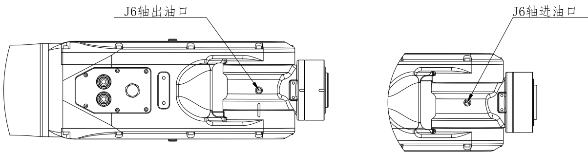
图 4-1 机器人注油口和排气口分布图
